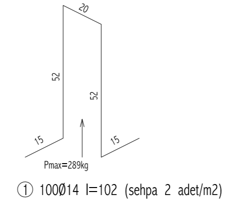
① 100Ø14 I=102 (setpa 2 adet/m 2 )
