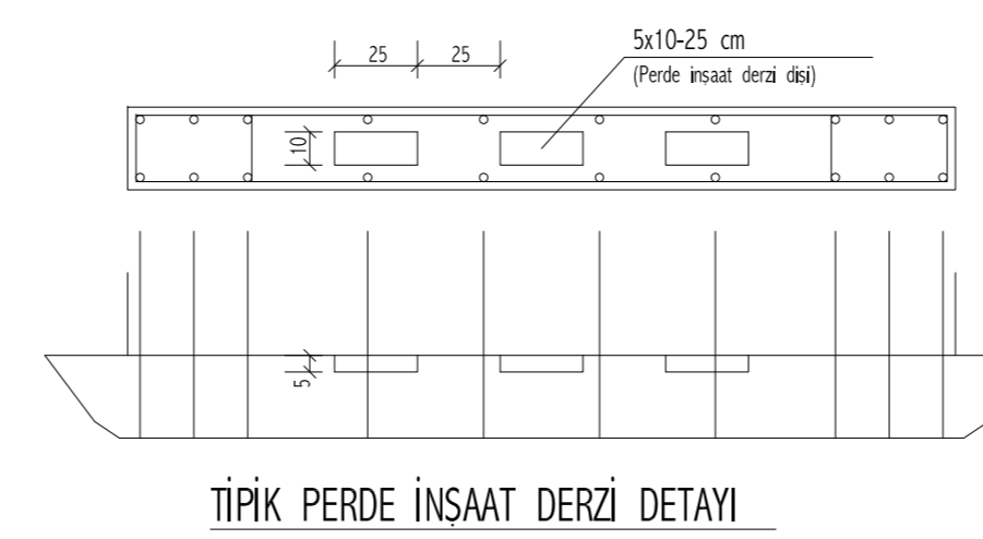
TİPİK PERDE İNŞAAT DERZİ DETAYI
