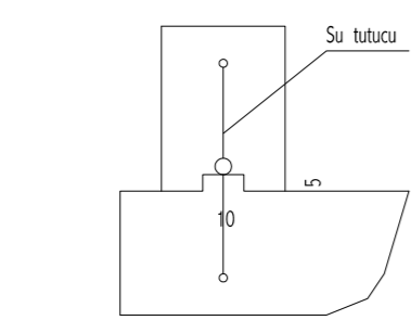
TİRKİ BODRUM PERDESİ İNŞAAT DERZİ DETAYI
